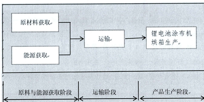
图 1 1 节锂电池涂布机烘箱碳足迹评价系统边界图
