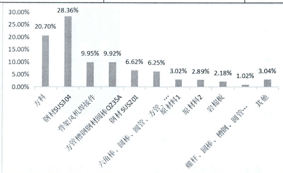
图 2 1 节锂电池涂布机烘箱产品原材料获取阶段碳足迹排放量占比
