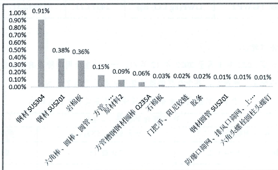
图 3 1 节锂电池涂布机烘箱产品原材料运输过程碳足迹排放量占比
